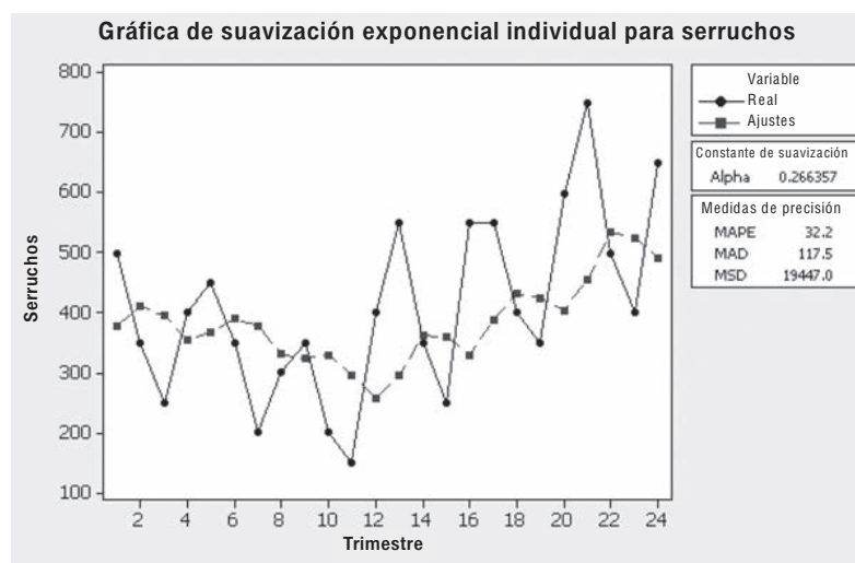
FIGURA 4-8 Suavización exponencial con \alpha = .266 para los datos de Acme Tool Company para el ejemplo 4.6
