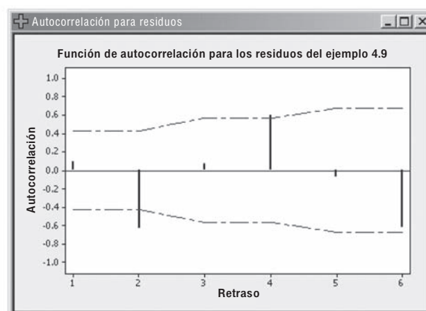
FIGURA 4-11 Función de autocorrelación de los residuos de la suavización exponencial lineal de Holt de los catos de Acme Tool Company para el Ejemplo 4.9
