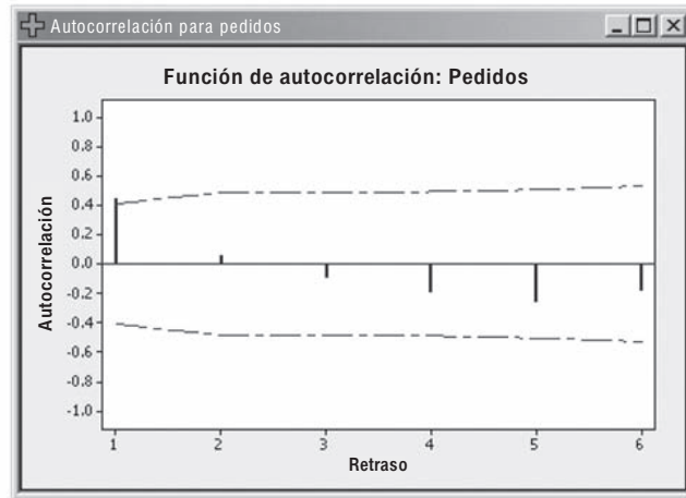
FIGURA 4-21 Función de autocorrelación para pedidos
