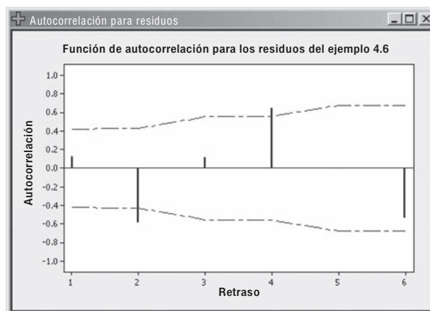
FIGURA 4-9 Función de autocorrelación para los residuos cuando se usa suavización exponencial con \alpha = .266 con datos de Acme Tool Company para el Ejemplo 4.6
