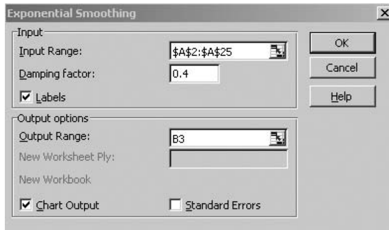
FIGURA 4-25 Ventana de diálogo de la Suavización exponencial de Excel
