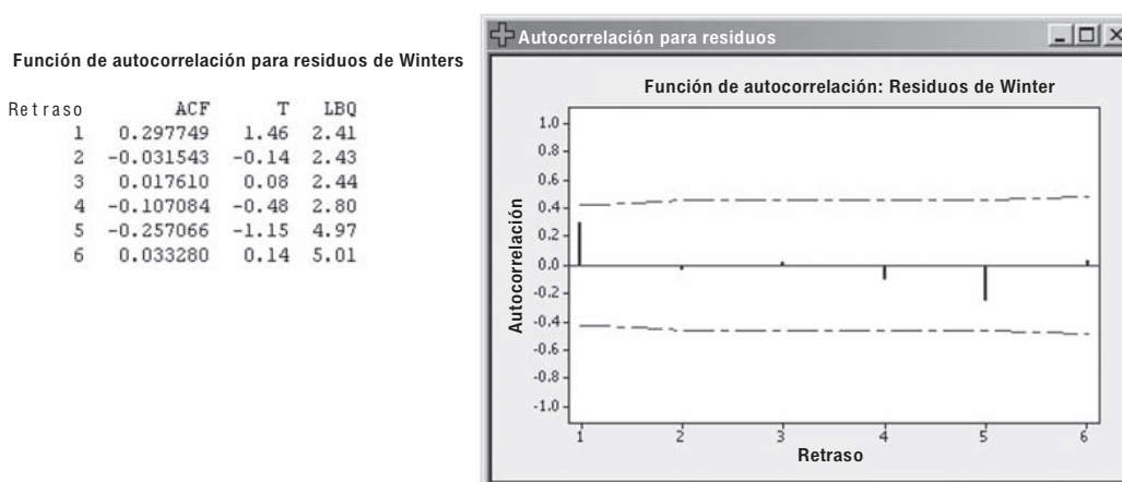
FIGURA 4-13 Función de autocorrelación del método de suavización exponencial multiplicativa de Winters de los residuos para los datos de Acme Tool Company para el ejemplo 4.10
