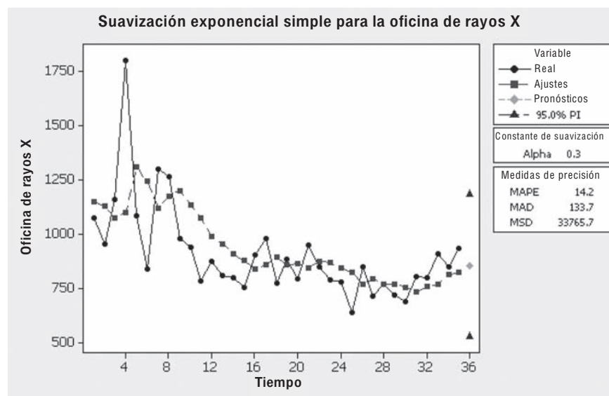
FIGURA 4-14 Suavización exponencial simple: Downtown Radiology, rayos X
