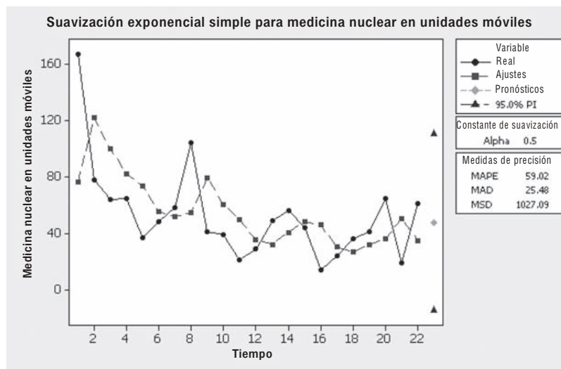
FIGURA 4-17 Suavización exponencial simple: Medicina nuclear en unidades móviles de Downtown Radiology
