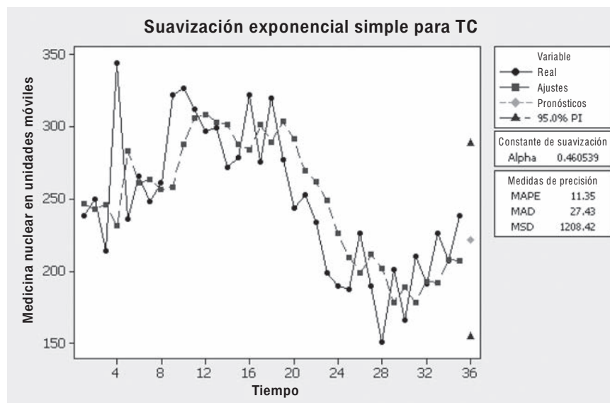
FIGURA 4-18 Suavización exponencial simple: Tomografías computarizadas de Downtown Radiology
